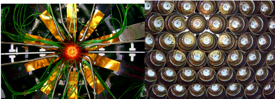
ALICE LHCb
