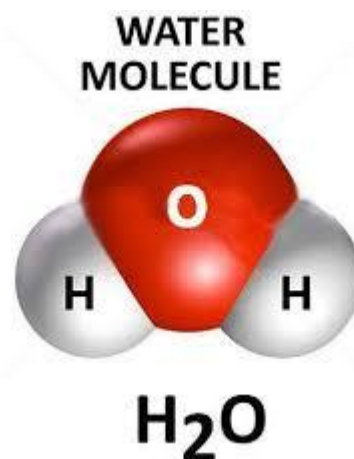
Молекула на водата
